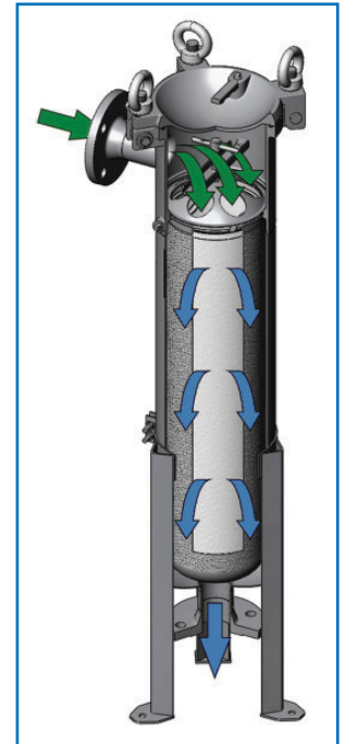
Durchfluss volume flow
