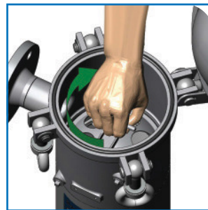
Andrückvorrichtung montieren mount filter bag fixing unit
