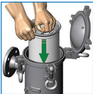
Filterbeutel einsetzen install filter bag
