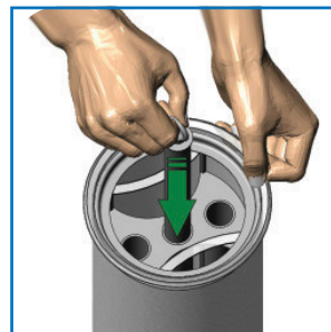
Magnetstab einführen (max. 3 Stk.) insert magnet bar (max. 3 pcs.)
