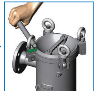
Ringmuttern anziehen tighten the ring nuts
