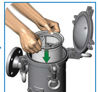
Filterbeutel einsetzen install filter bag
